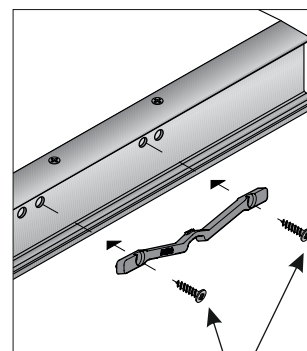
Шуруп 3,5*25 мм
