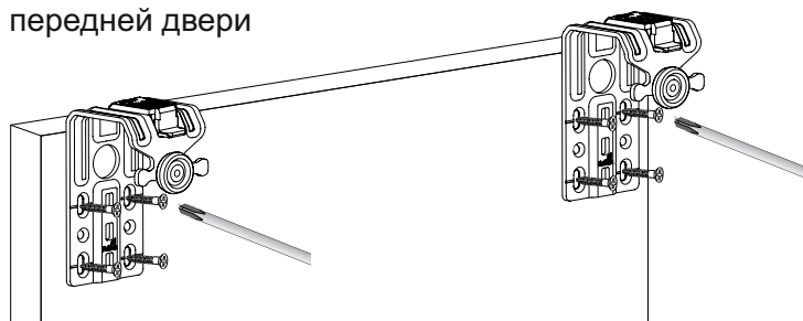
Монтаж ходового элемента для задней двери
