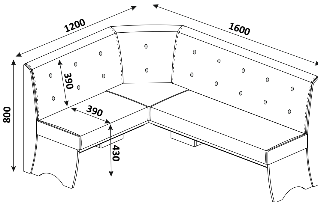
Скамья угловая
