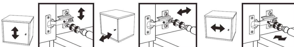
Схема регулировки двери:
